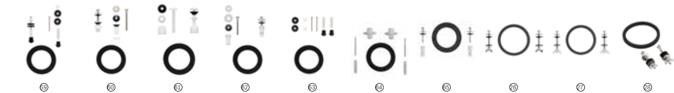
Fijaciones y junta taza-tanque
